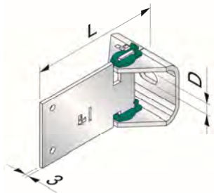
L = Schwert mit Konsole
