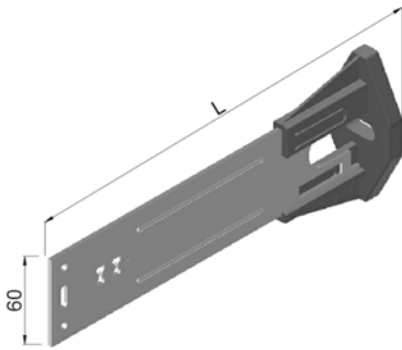
L = Schwert mit Konsole
