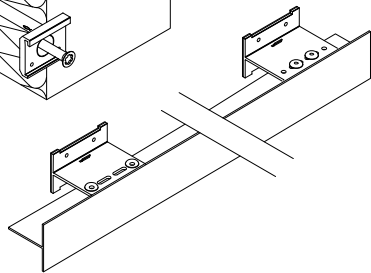
Horizontale Tragprofile
