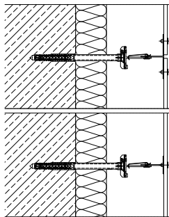
Horizontale Tragprofile
