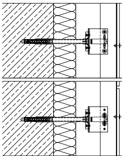
Vertikale Tragprofile
